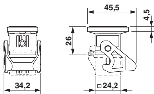
尺寸图
