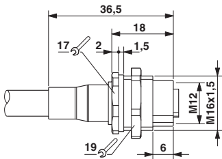
尺寸图
