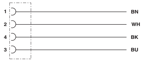
电路图
