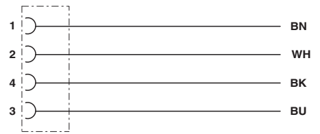
电路图
