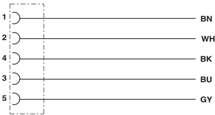
电路图
