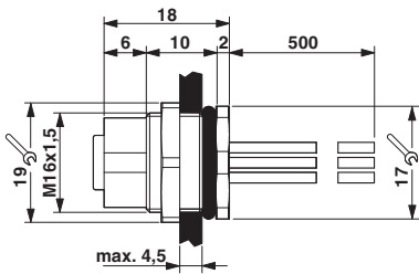
尺寸图
