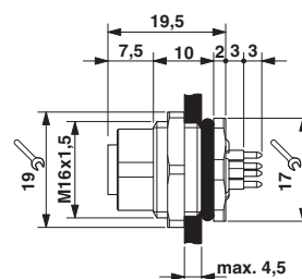
尺寸图
