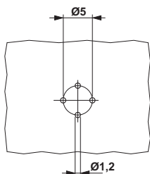
钻孔图
