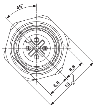
尺寸图
