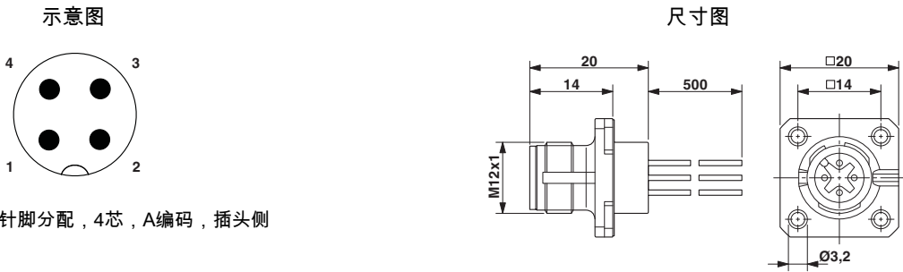
M12穿板式插头，方方法兰
