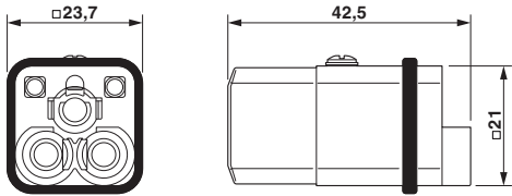
尺寸图
