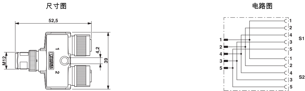
M12 Y型分配器的触点分配
