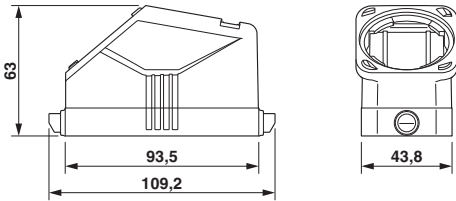
尺寸图
