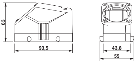
尺寸图
