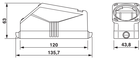
尺寸图
