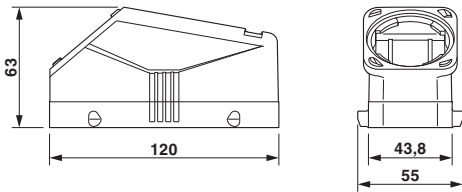
尺寸图
