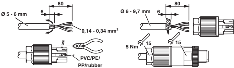
功能图
