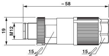
尺寸图
