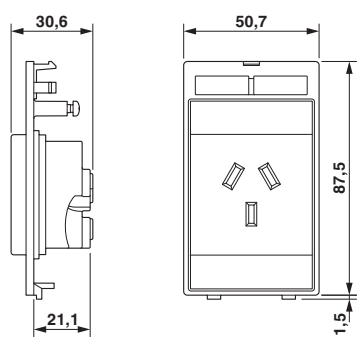
尺寸图
