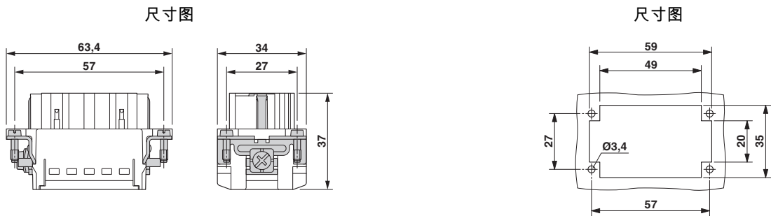
不使用外壳时的安装开口
