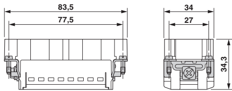
尺寸图
