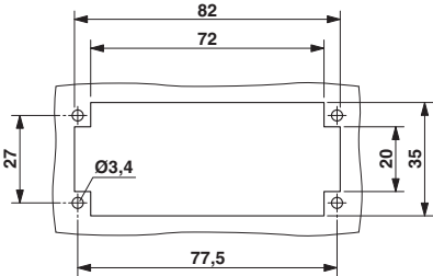
尺寸图
