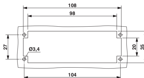
尺寸图
