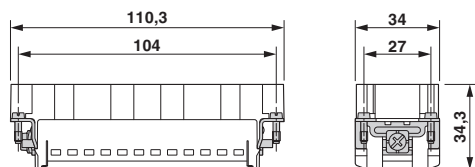
尺寸图
