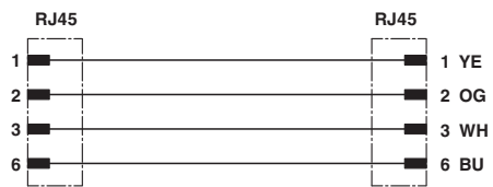
电路图
