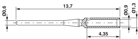
尺寸图
