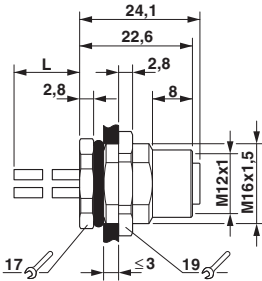
尺寸图
