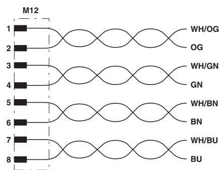
电路图
