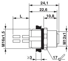
尺寸图
