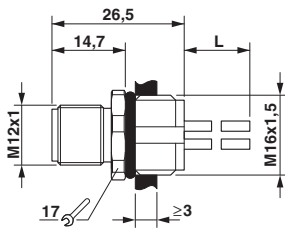
尺寸图
