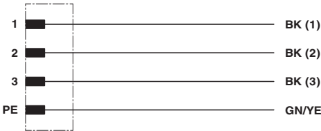
电路图
