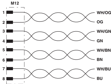
电路图
