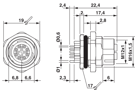
尺寸图
