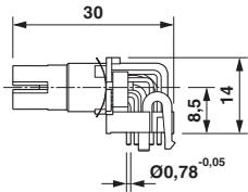
尺寸图
