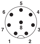
M8针式连接器引脚分配，8芯，插头侧视图
