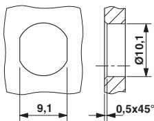
尺寸图
