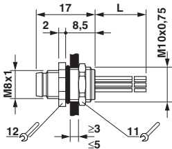
尺寸图
