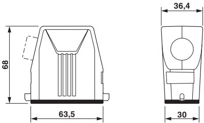
尺寸图
