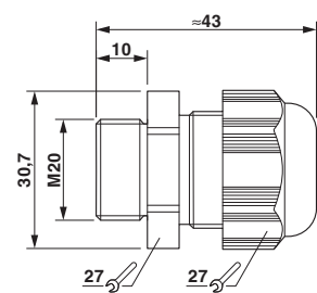
尺寸图
