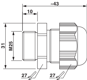
尺寸图
