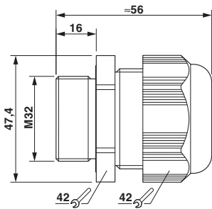
尺寸图
