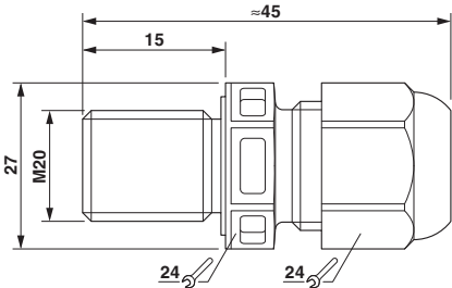
尺寸图
