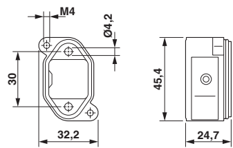
尺寸图
