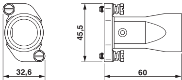
尺寸图
