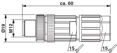
尺寸图
