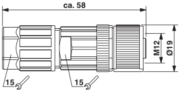
尺寸图
