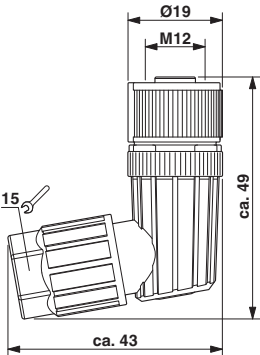
尺寸图
