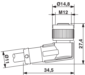
尺寸图
