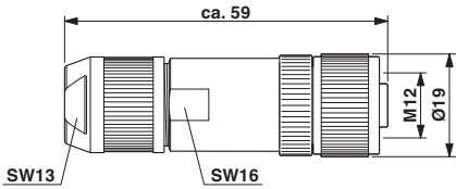
尺寸图
