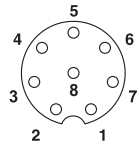
M12孔式接头的引脚分配，6芯，插座侧视图
