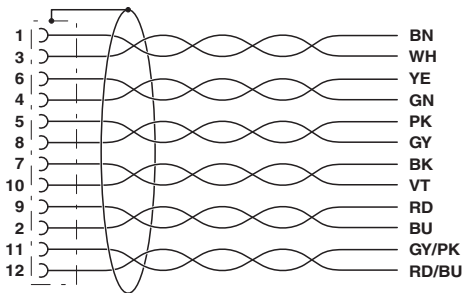
电路图
