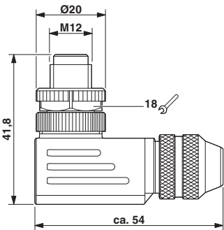
尺寸图
