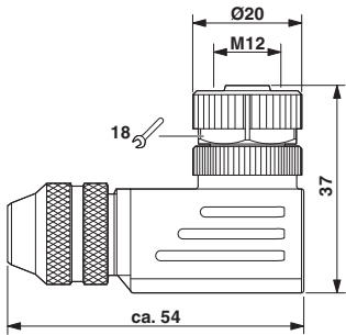
尺寸图
