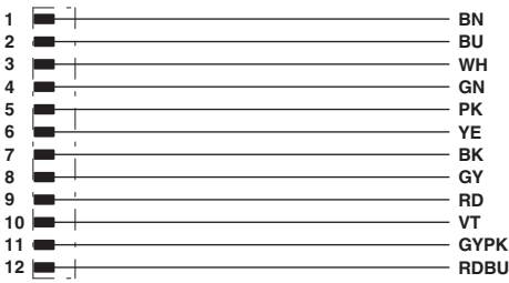
电路图
