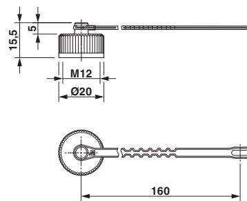
尺寸图
