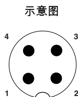
M12针式连接器引脚分配, 4芯, A编码, 插头侧视图
