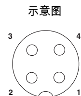
M12孔式连接器引脚分配, 4芯, A编码, 插座侧视图
