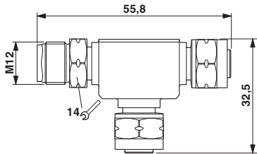
尺寸图
