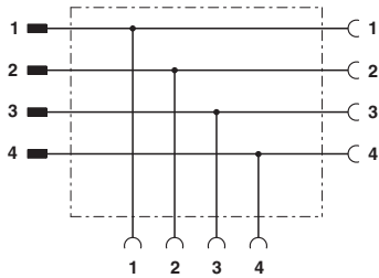
电路图
