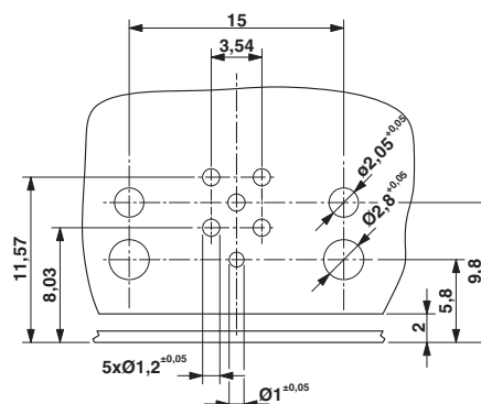
钻孔图
