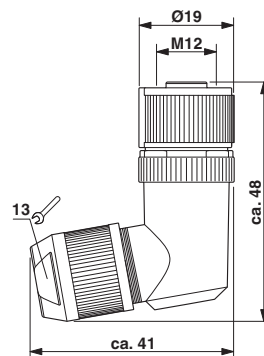
尺寸图
