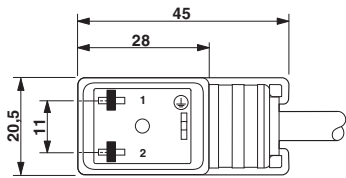
尺寸图
