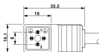
尺寸图
